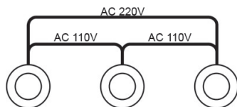
Modelo monofásico
