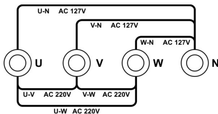
Modelo trifásico 220V
