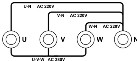
Modelo trifásico 380V
