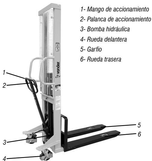
Fig. 1 - Componentes
