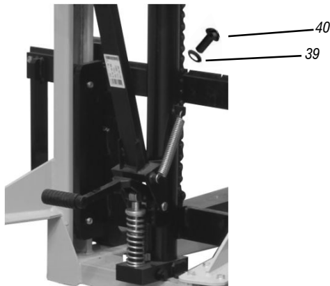
Fig. 6 Completando/Substituyendo el aceite
